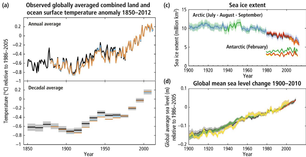
Impacto das alterações climáticas, observado durante o último século, na subida média da temperatura, no decréscimo dos glaciares e no aumento do nível do médio do mar.
