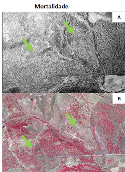
A) 1979 - floresta densa de sobreiro e de azinheira; B) 2018 - área de montado e/ou área agrícola, após a mortalidade de grande parte do arvoredado. Setas apontam áreas notáveis
